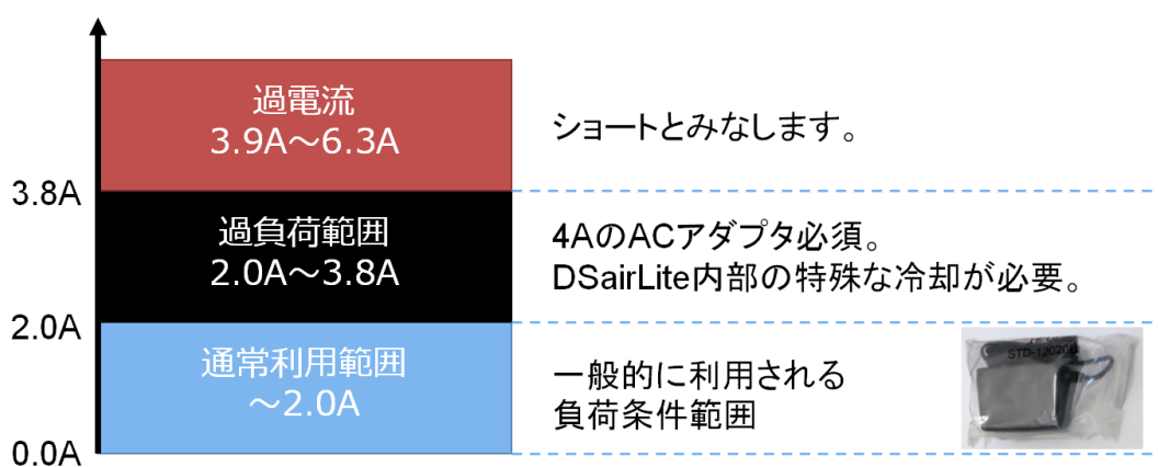
図 2.2 DSairLite の消費電流と負荷範囲
