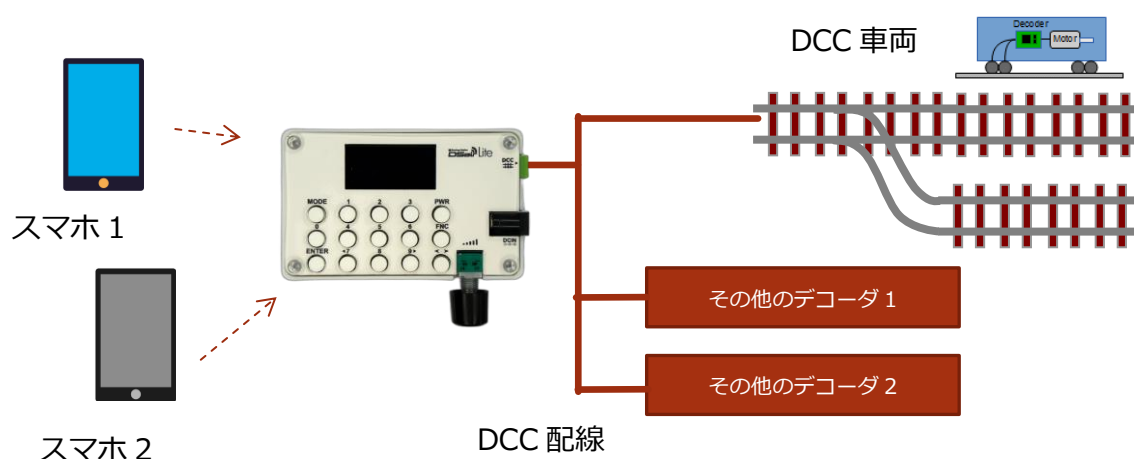
図 5.1 Web アプリを用いた WiFi による DSairLite の遠隔操作構成例
