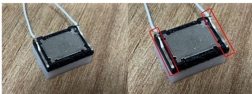
図 5.9.1 キューブスピーカーの導電部
