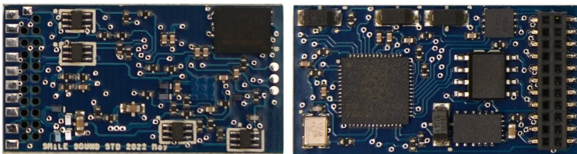
図 5.5.1.1 SmileSound Standard MTC21 の外観
