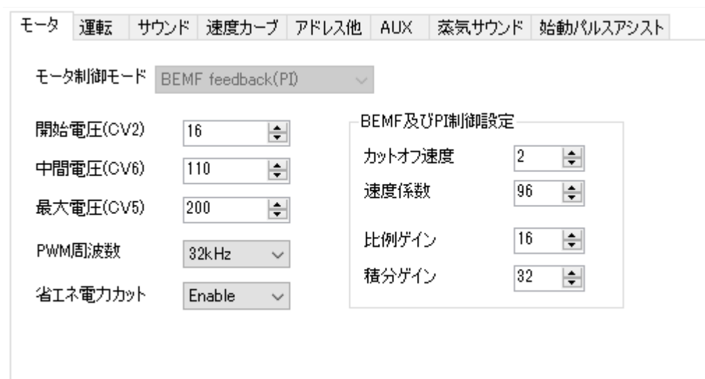
図 9.3.1 モータ CV 設定画面
