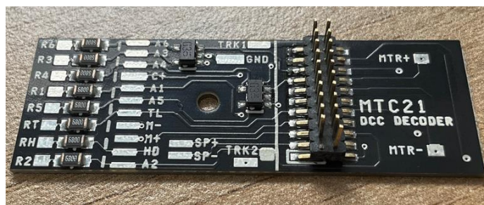
図 5.4.6.2 10047/10050 ExpBoard M21 Super Short 幅狭版
