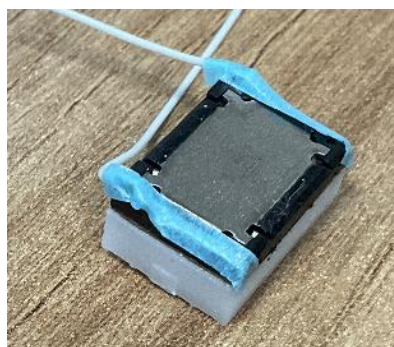
図 5.9.3 マスキングテープで絶縁対策したスピーカー
